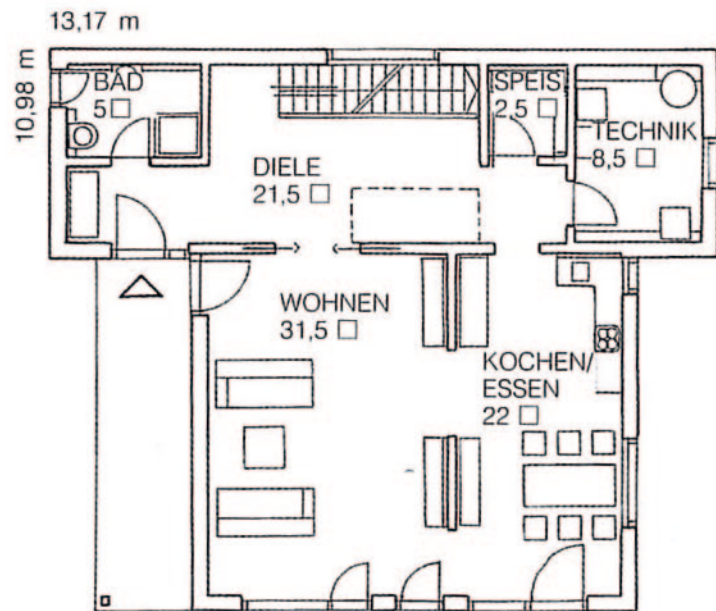
ERDGESCHOSS
